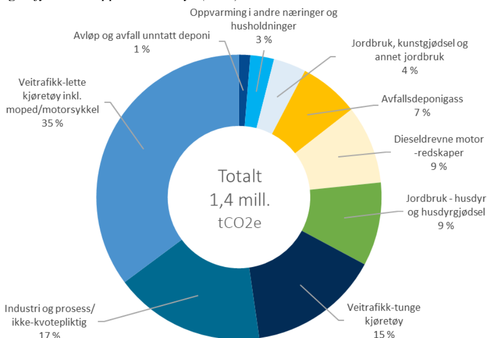
Figur 1: Direkte utslipp fra ikke-kvotepliktig sektor i Agder, 2015. Kilde: Klimaregnskap for Agderfylkene, Rapport CEMAsys (2017)
